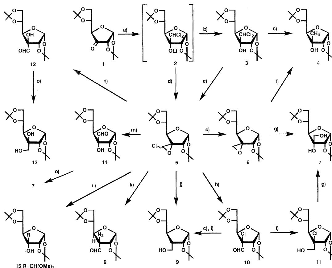
Scheme 2. a) LDA, \text{CH}_2\text{Cl}_2 , oxolane, -78^\circ\text{C} b) \text{H}_2\text{O} , r.t. c) n\text{-Bu}_3\text{SnH} , AIBN, toluene, reflux. d) 65^\circ\text{C} . e) DBU, DMSO, r.t. f) \text{LiAlH}_4 , oxolane, r.t. g) \text{NaOH} aq, 1,4-dioxane, reflux. h) \text{NaOAc} , 15-crown-5, HMPT, 70^\circ\text{C} . i) \text{NaBH}_4 , aq MeOH, r.t. j) \text{NaBH}_4 , DMSO, 80^\circ\text{C} . k) \text{NaN}_3 , 15-crown-5, HMPT, 70^\circ\text{C} . l) \text{NaOMe} , HMPT, 70^\circ\text{C} . m) n\text{-Bu}_4\text{NOH} aq, DMSO, r.t. n) \text{CsOAc} , 18-crown-6, toluene, reflux. o) \text{NaBH}_4 , MeOH, r.t.
